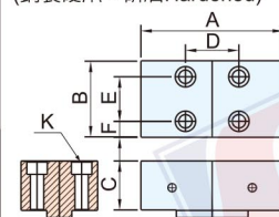
Movable Jaw / 活動口金 (鋼製硬爪, 研磨 Hardened)
