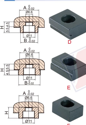
壓塊固定圖 Clamp kits
