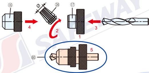
B. 如何完成鑽頭長度及方位設定之準備
